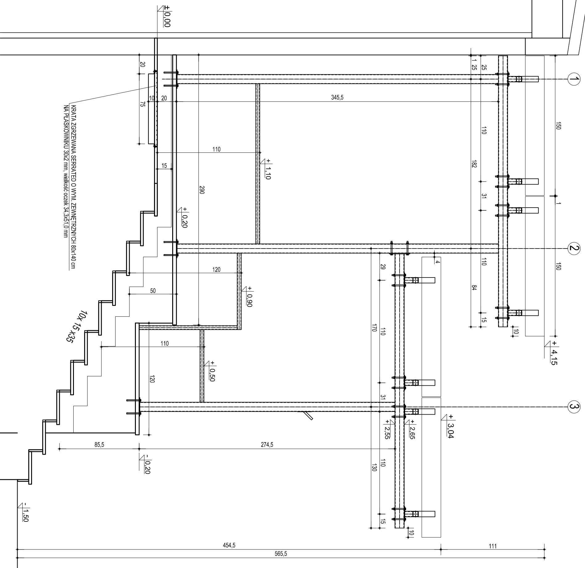
RYS. NR 5 PRZEKRÓJ A-A - stan projektowany SKALA 1 : 25
