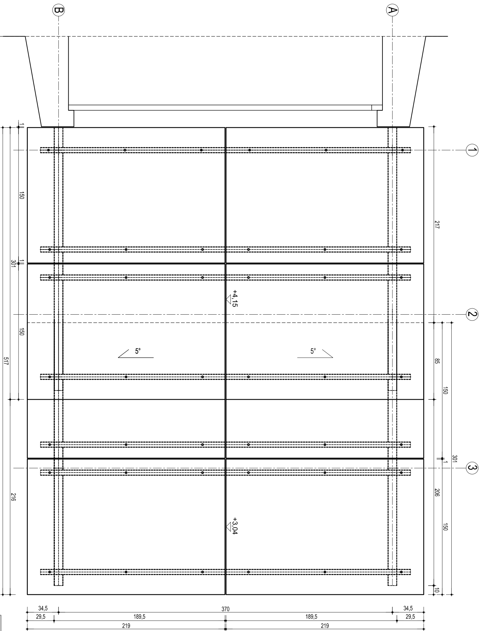
RYS. NR 4 RZUT DACHU - stan projektowany SKALA 1 : 25
